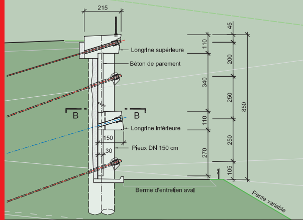
Coupe type A-A (zone centrale)
